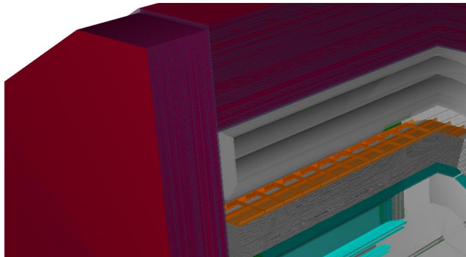
HcalBarrelClusters.energy
