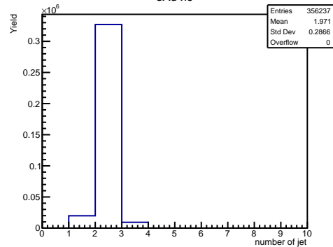
eAu nc
