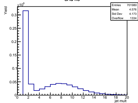
eAu nc
