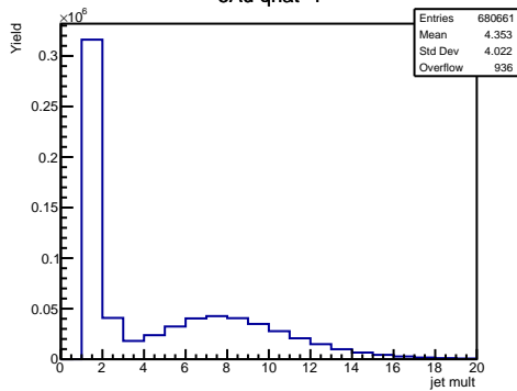
eAu qhat=1
