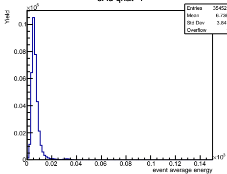
eAu qhat=1
