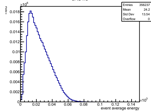
eAu nc
