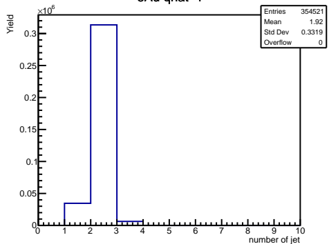
eAu qhat=1
