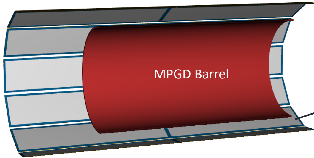
MPGD DIRC
