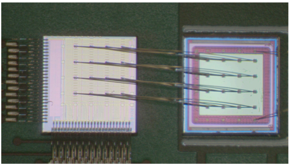
EICROC0 AC-LGAD
