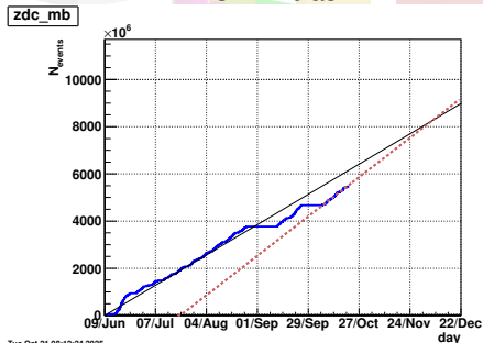
ZDC min-bias
