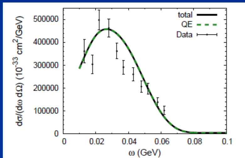
0.24 GeV, 36 deg, Q^2 = 0.02 \text{ GeV}^2
