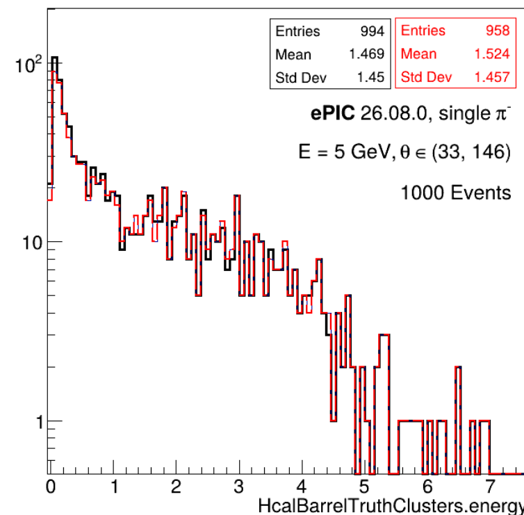
HcalBarrelTruthClusters.energy
