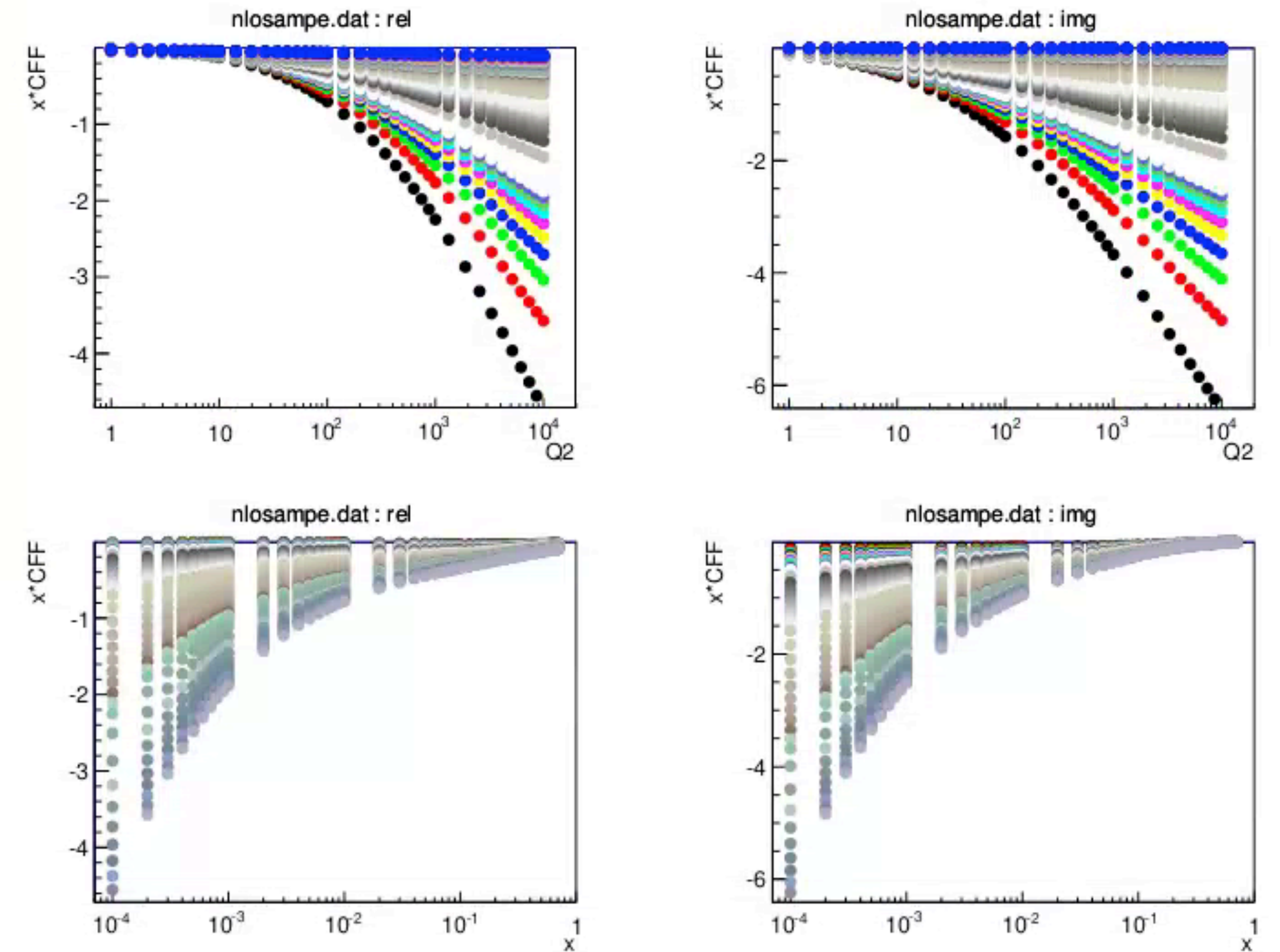
PARTONS
