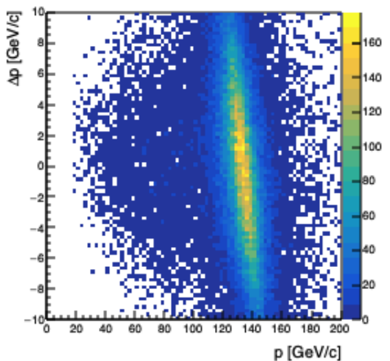
neutron_delta_p_vs_p
