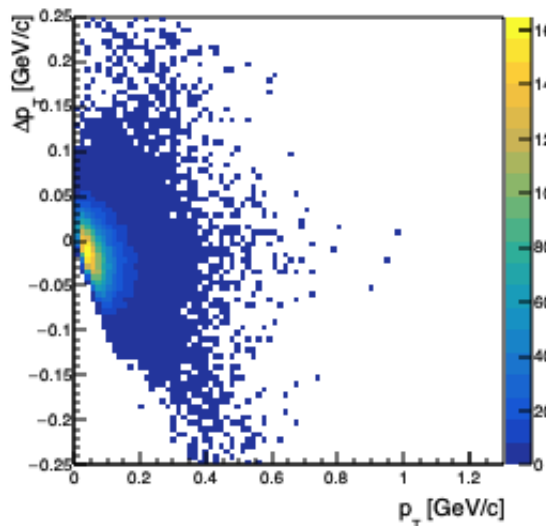
neutron_delta_pt_vs_pt
