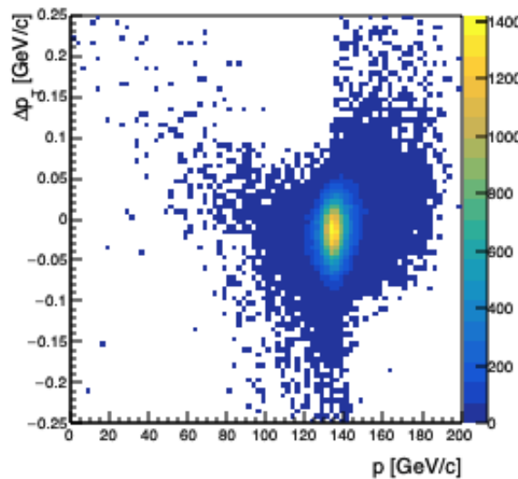
neutron_delta_pt_vs_p
