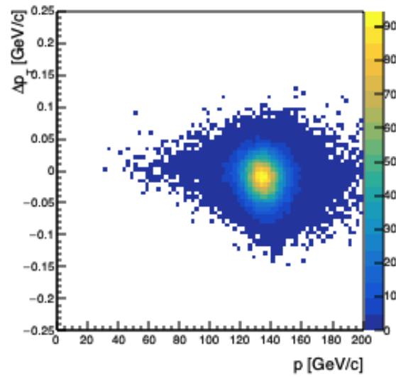
neutron_delta_pt_vs_p
